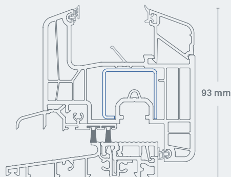
Nowość : Bezbarierowy próg do drzwi balkonowych Rys.: 1:2
