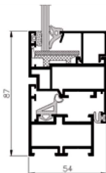
przekrój okna
