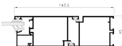
przekrój drzwi
