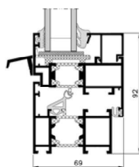
przekrój okna
