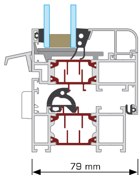
przekrój okna
