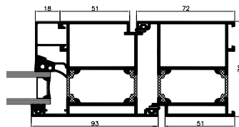
przekrój przez drzwi
