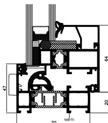
przekrój okna otwieranego
